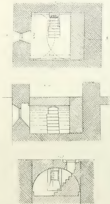
Fig. 30. Plan i przekroje podziemia wieży południowej.
